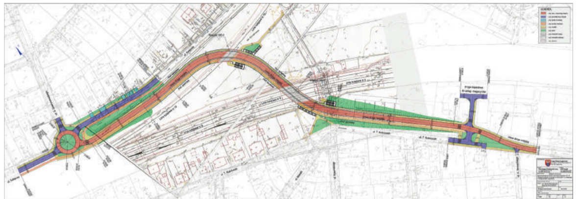
▲ Projekt pierwszej przeprawy w ul. Krasieńskiego
